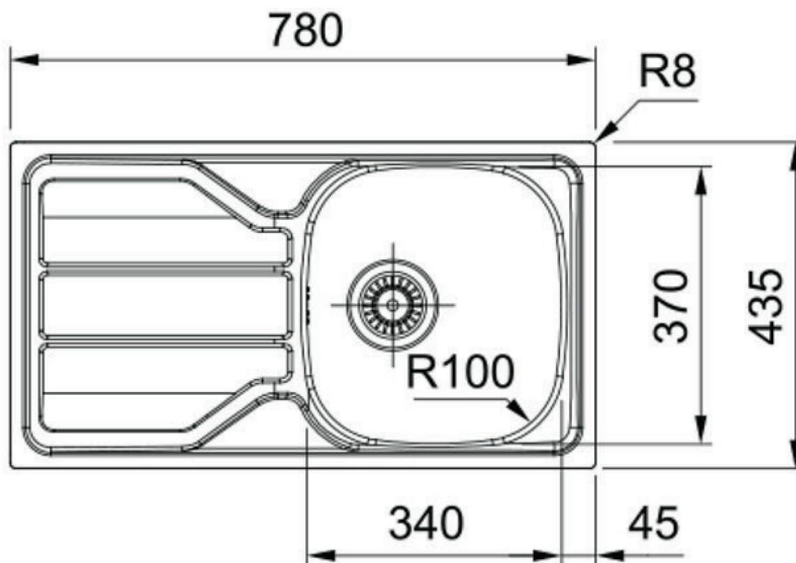
Modèle 1 cuve
